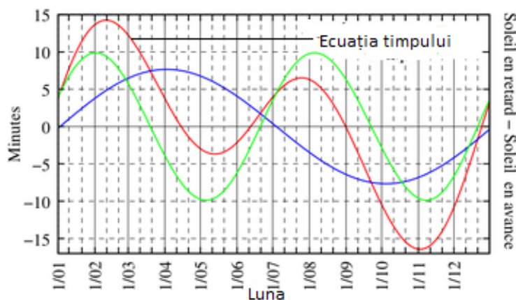
Figura 1. Ecuația timpului în funcție de data din an.
