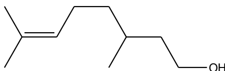
II. citronelol
