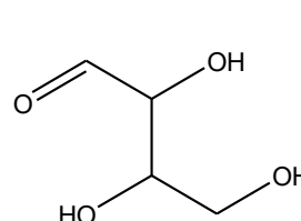
III. aldotetroză
