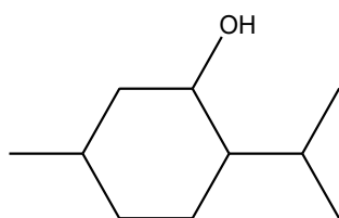
I. mentol
